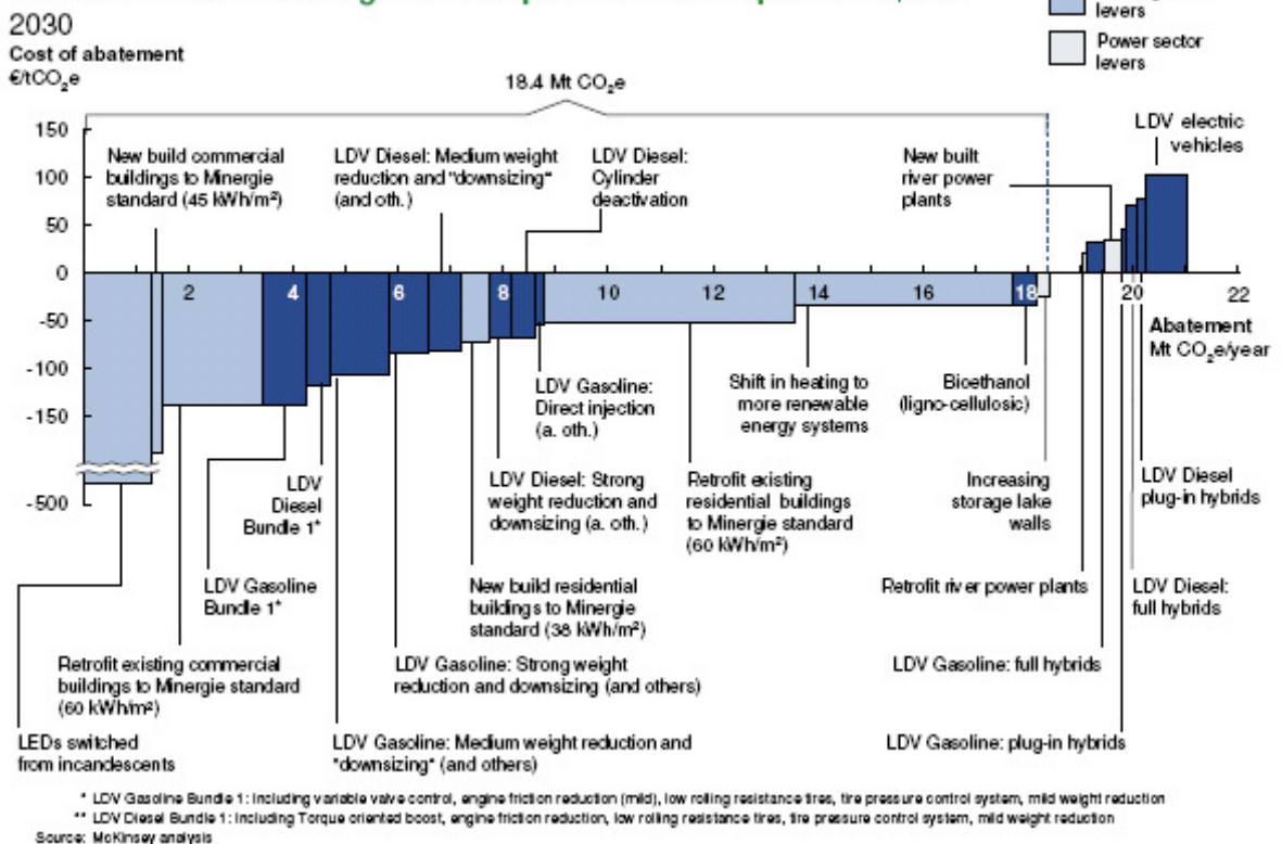
Fig.1: Geordnete Grenzkostenkurve für Klimaschutzmassnahmen in der Schweiz (McKinsey 2009, http://www.mckinsey.com/client/service/ccsi/pdf/GHG_cost_curve_report_final.pdf )
