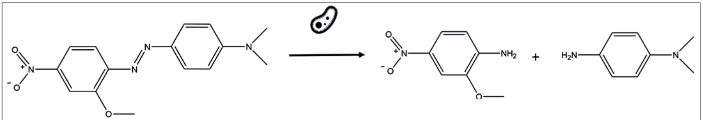
Spaltung des Azofarbstoffs Dispersionsrot 41 (CAS-Nr. 6373-90-6) bei der Azobindung (rot markiert) durch Bakterien in zwei aromatische Amine. Das linke aromatische Amin ist 2-Methoxy-4-nitroanilin (CAS-Nr. 97-52-9) und wirkt mutagen.
