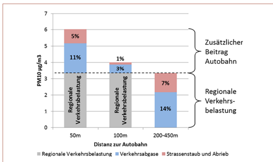
Durchschnittliche Zusatzbelastung durch verkehrsbedingten Feinstaub (PM10) von der Autobahn in Erstfeld (UR), in Prozent des total gemessenen Feinstaubes. (Quelle: Schweizerisches Tropen- und Public Health-Institut 2 )
