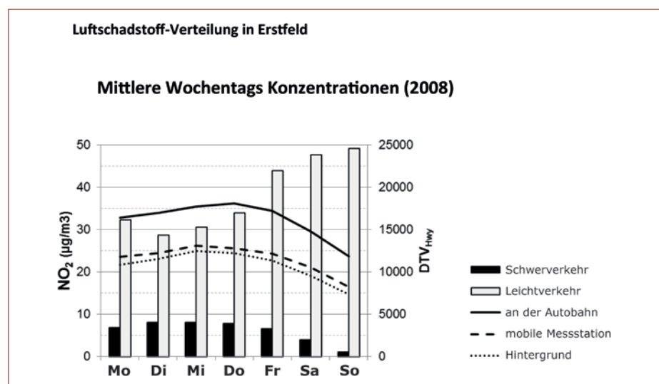
Einfluss des Autobahnverkehrs auf die Luft in Erstfeld (UR). Die Stickstoffdioxid-Konzentrationen folgen dem Verlauf des Schwerverkehrsaufkommens. Mittlere Wochentags-Konzentrationen 2008. DTV = durchschnittlicher Tagesverkehr. (Quelle: Ducret-Stich et al., Sci Total Environ 2013).
